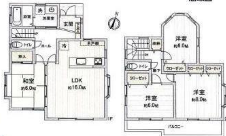
間取図
