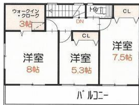
2階平面図 S: 1/120
